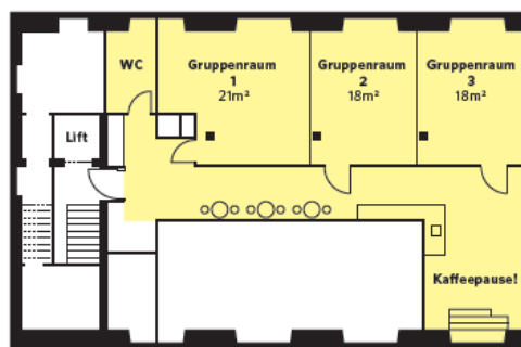
Grundriss UG
